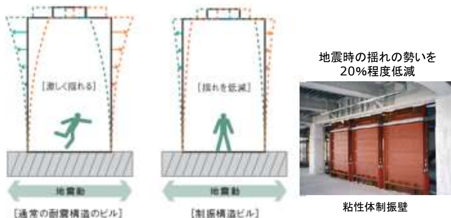
制振構造
