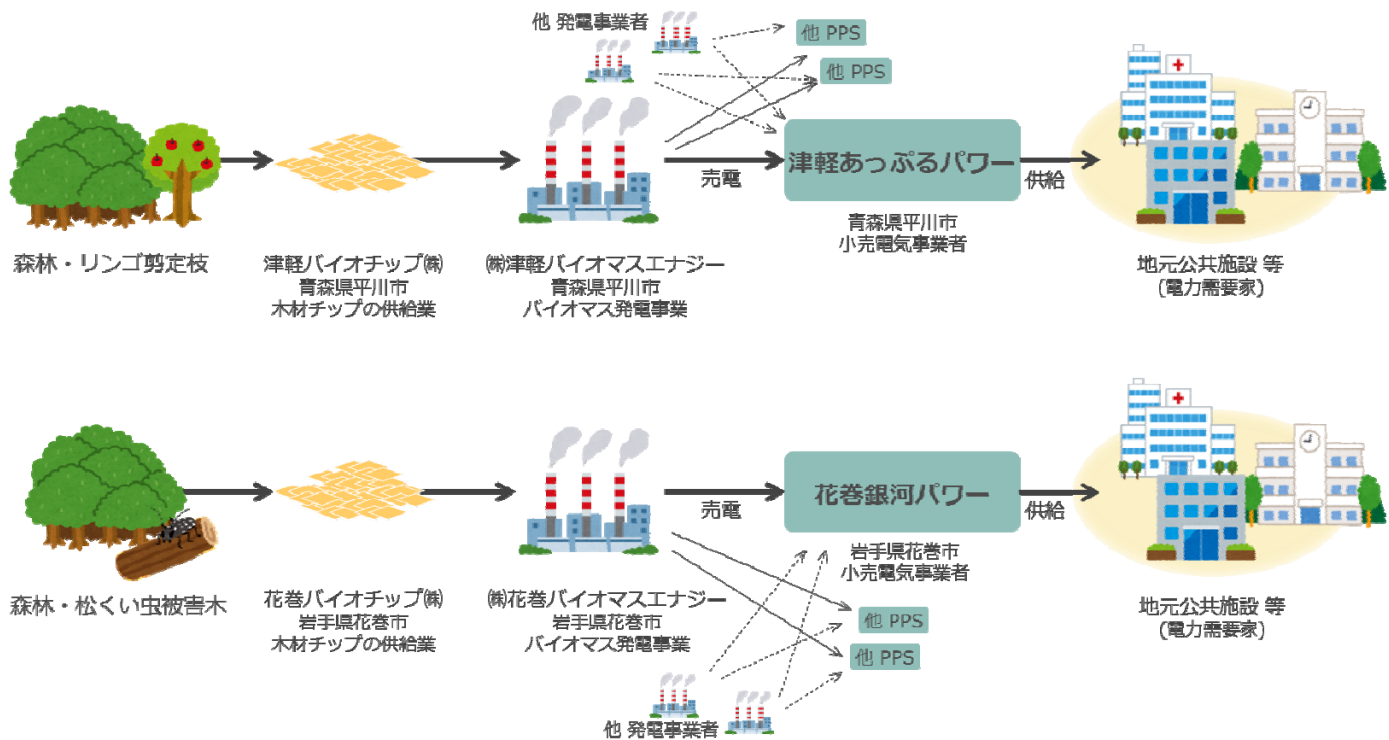
図1. 電力の地産地消 スキーム
