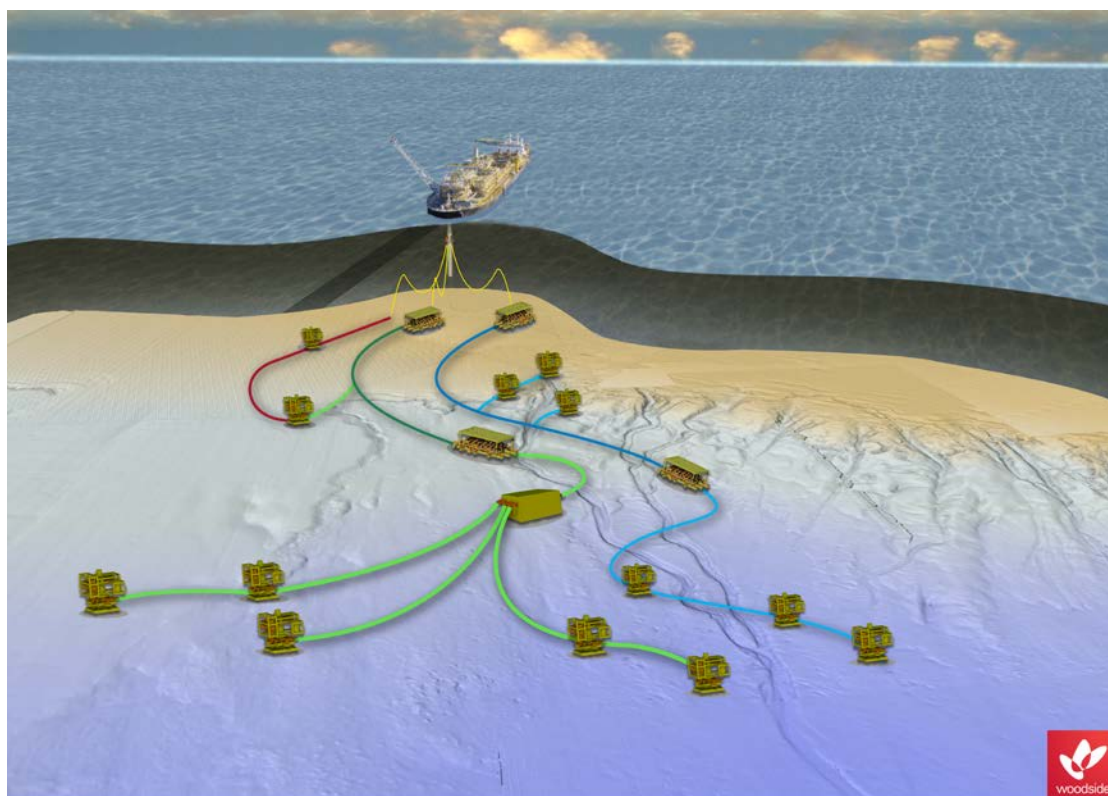
グレーターエンフィールドプロジェクト：ヴィンセント油田で使用する Ngujima-Yin FPSO へ海底で繋ぎ込む。画像は Woodside 提供。
