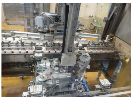
箱詰めロボット
