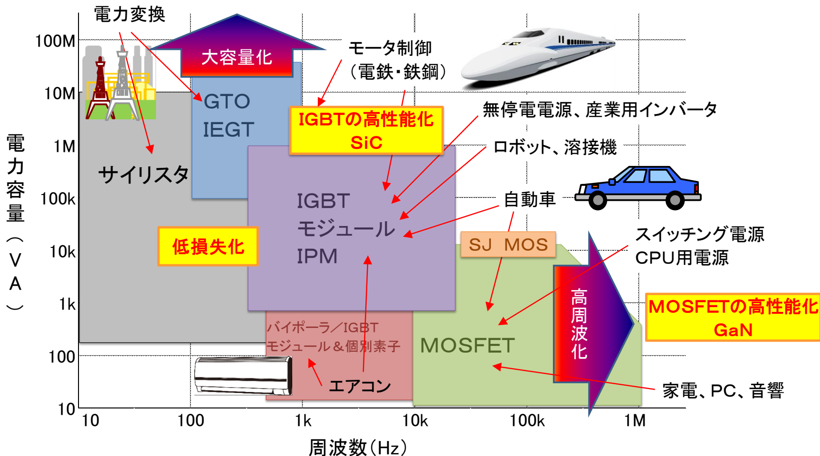
パワーデバイスの種類とアプリケーション
