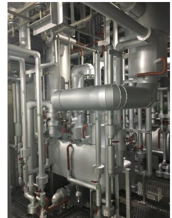
連続蒸留設備写真(一部)
