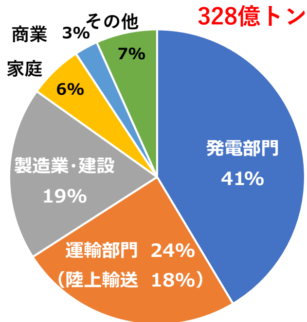
世界の部門別CO 2 排出量（2017年）
