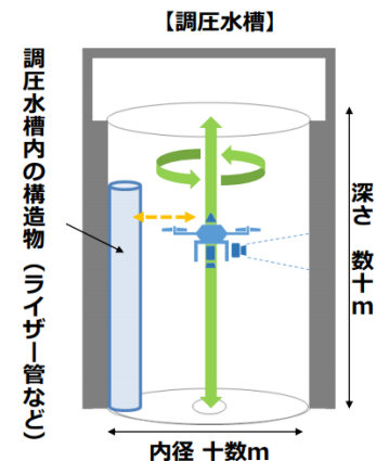
▲調圧水槽内を降下しながら壁面を撮影するドローン
