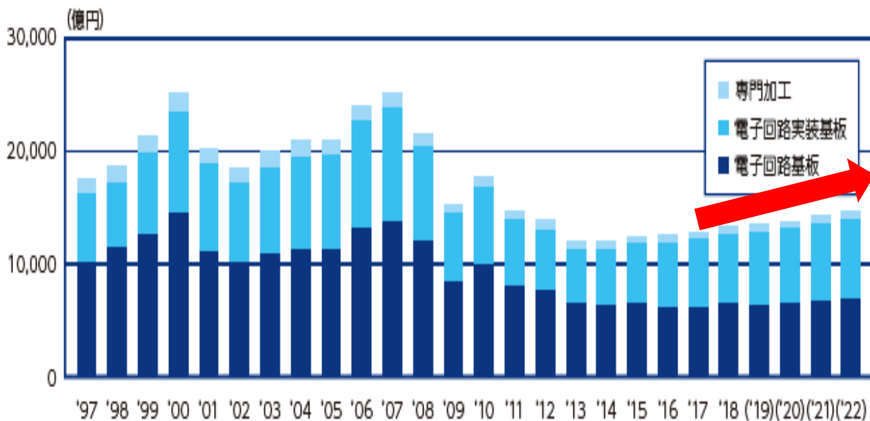
国内の電子回路の製造区分別の生産推移と将来予測
