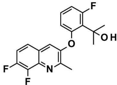
日本曹達が開発した新規殺菌剤キノプロール（製品名「ミギワ」）の構造式 2-[2-(7,8-difluoro-2-methylquinolin-3-yloxy)-6-fluorophenyl]propan-2-ol
