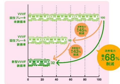
VVVFインバータ制御装置更新 による消費電力削減効果
