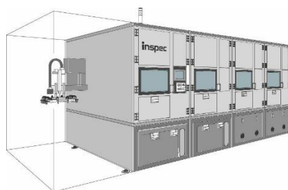
AI機能付両面全自動検査装置イメージ図
