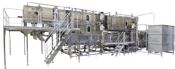
CIP自動茹麺装置
