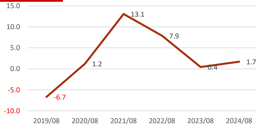
ROE(%)
