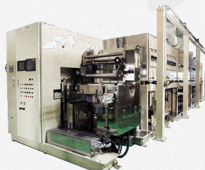
▲ Li電池・電極用コーター R-800DB
