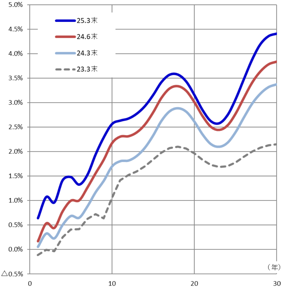
フォワード・レート（23.3-25.3）
